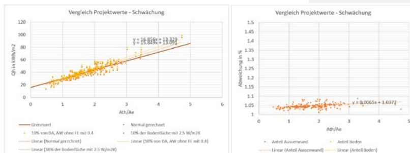
Figura 14: Confronto tra la retta di regressione ENteb "normale" di una casa monofamiliare con quella dello stesso progetto ma con il 10% della superficie di elementi opachi con valori U di 0.4 W/(m²·K). Risultato: circa 5% di maggior fabbisogno termico di riscaldamento.
