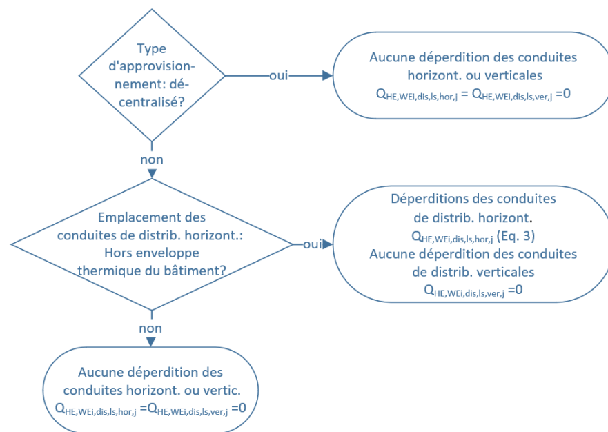
Ill. 3 Diagramme de flux – Déperditions liées à la distribution du chauffage.
