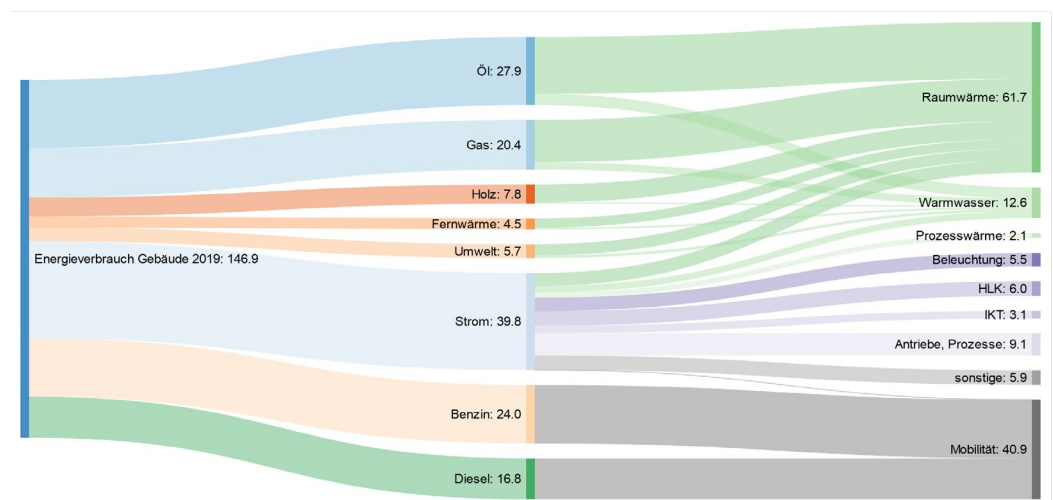
Abb. 4 Consommation d'énergie par type d'utilisation et agent énergétique Situation en 2019 [TWh]
