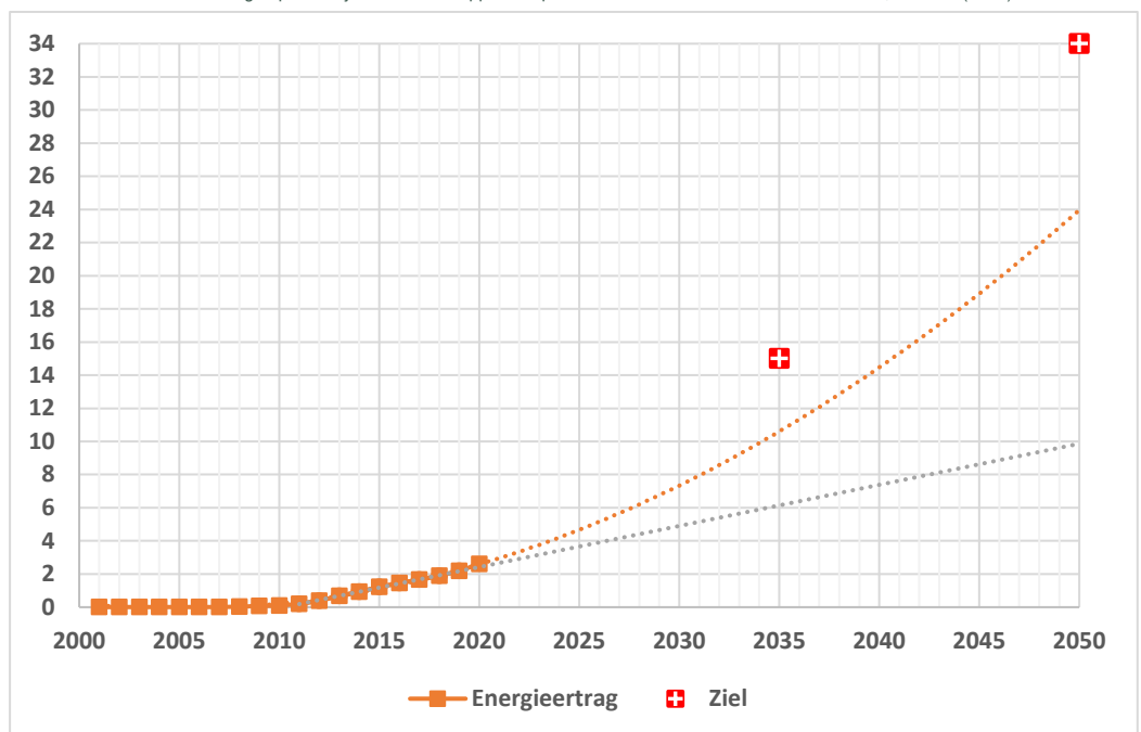
Abb. 10 Rendement énergétique et objectifs de développement pour les installations PV installées en Suisse, en TWh (2021)
