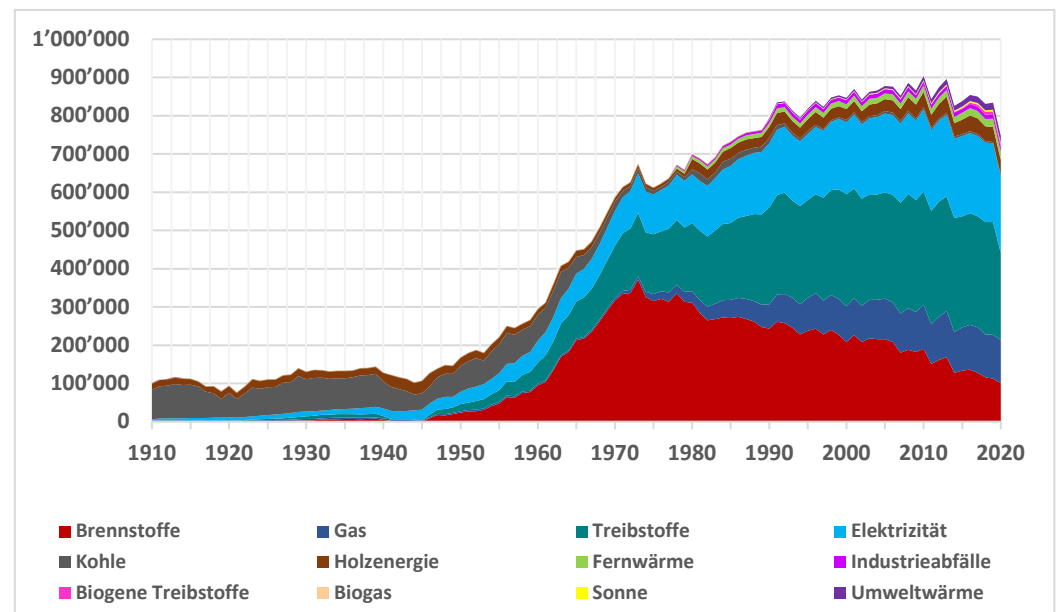
Abb. 2 Consommation finale d'énergie 1910-2020, par agent énergétique [TJ]
