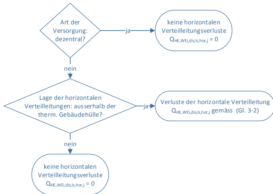
III. 3 Diagramme de flux – Déperditions liées aux conduites de distribution horizontales pour le chauffage ( Q_{HE,WE,dis,ls,hor,j} ).
