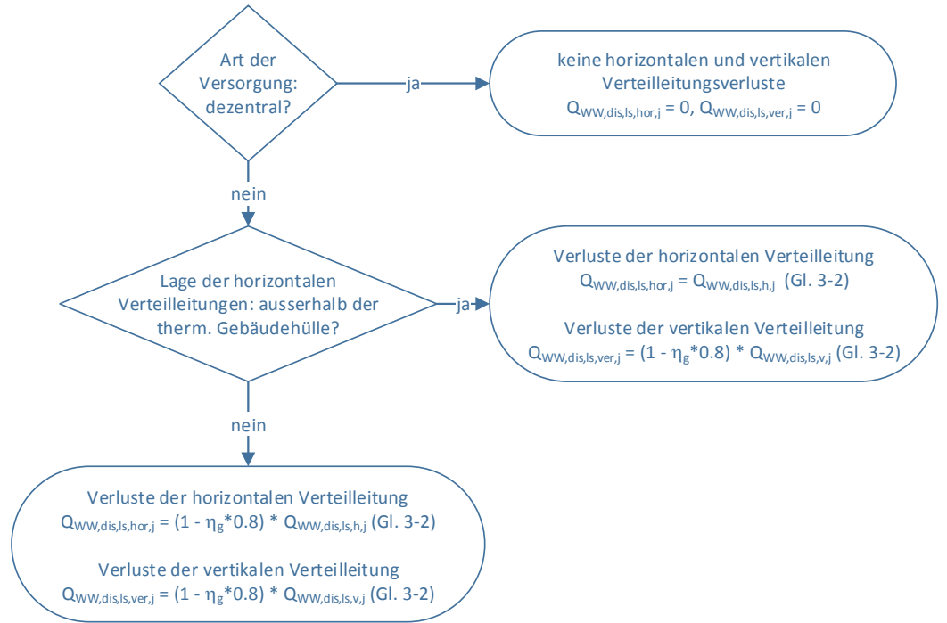
III. 4 Diagramme de flux – Déperditions liées aux conduites de distribution horizontales et verticales pour l'eau chaude.
