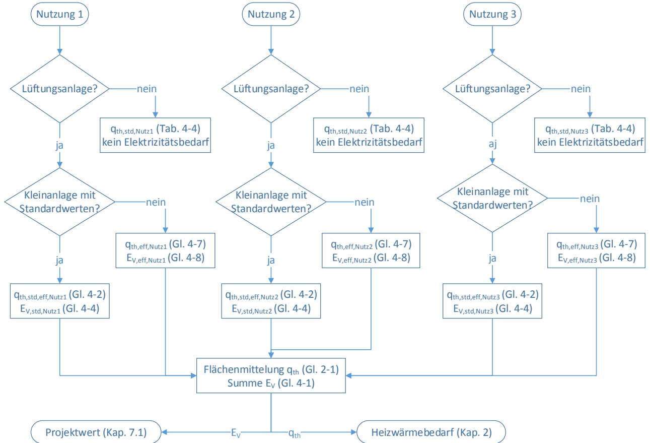
III. 5 Diagramme de flux – Calcul des débits d'air neuf actifs effectifs et des besoins en électricité.
