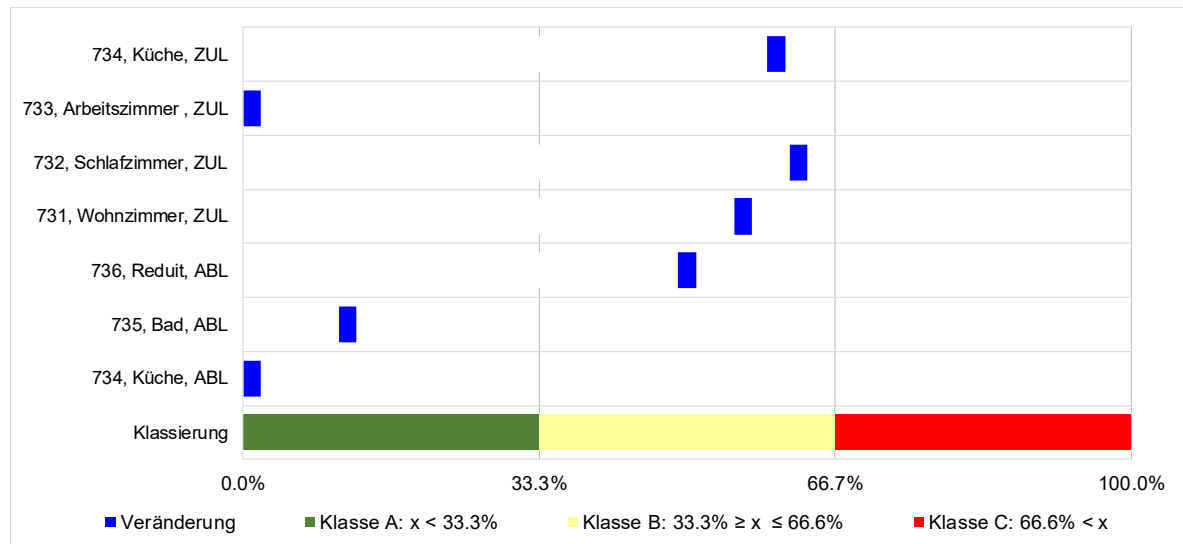
Abbildung 162: Wohnung ID 730: Veränderung der Luftmengen vor / nach der Reinigung bzw. Filterersatz
